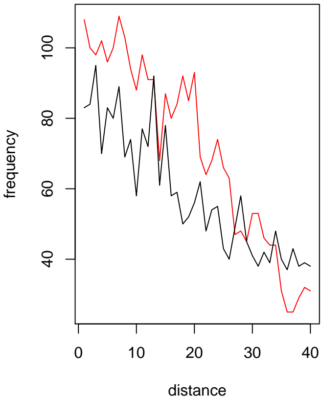
CTCF & Rad21
