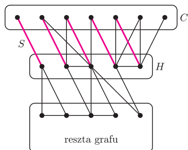
Rys. 2. Rozkład koronny grafu G .
