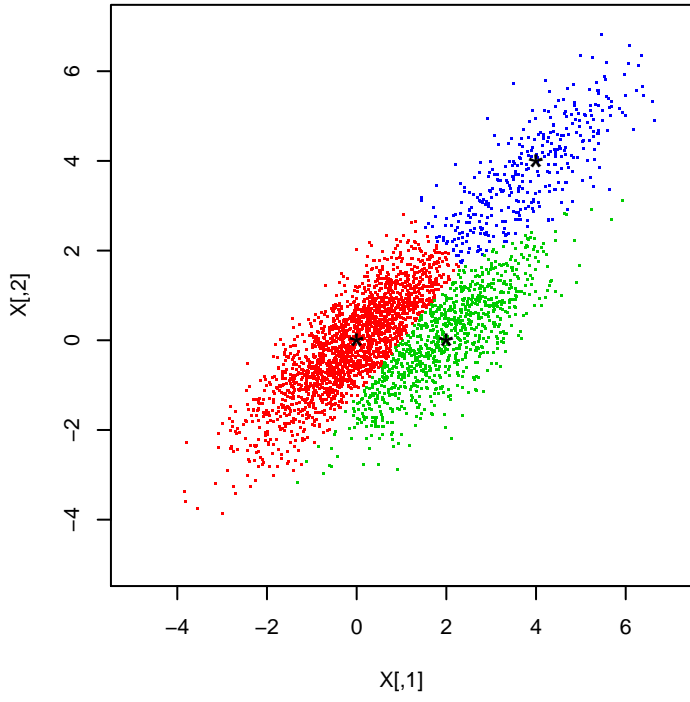
klasyfikacja optymalna
