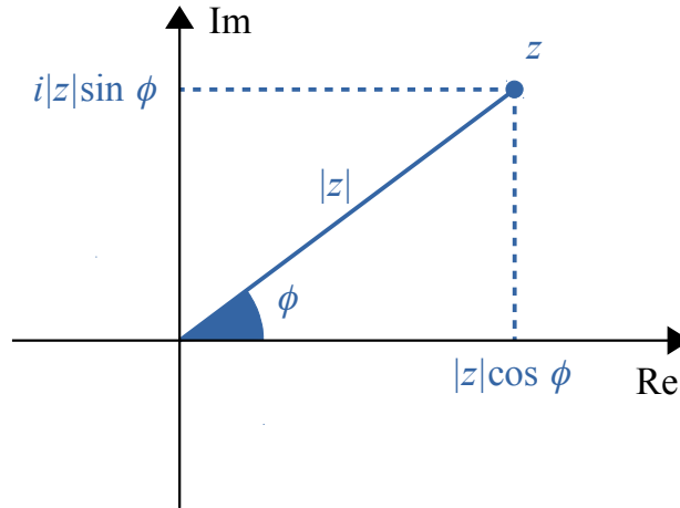
Rysunek 2.3: Postać trygonometryczna liczby zespolonej
