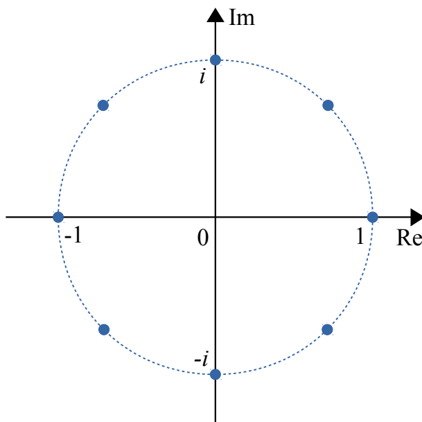
Rysunek 2.5: Pierwiastki z jedności stopnia 8
