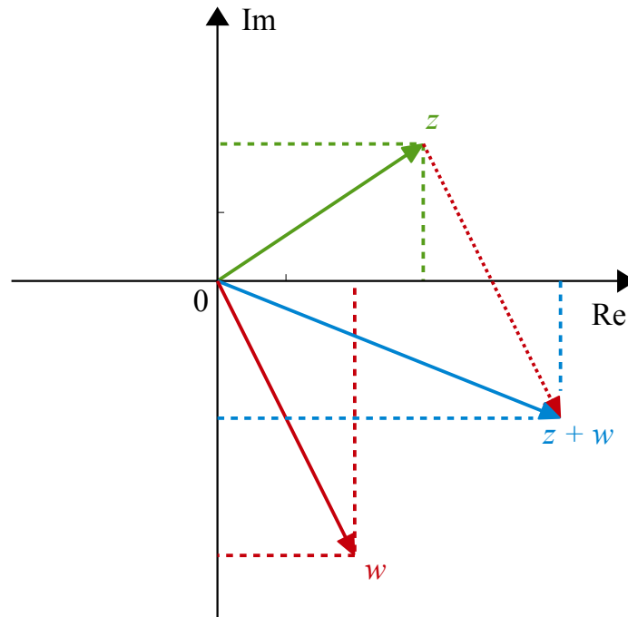
Rysunek 2.2: Dodawanie liczb zespolonych.
