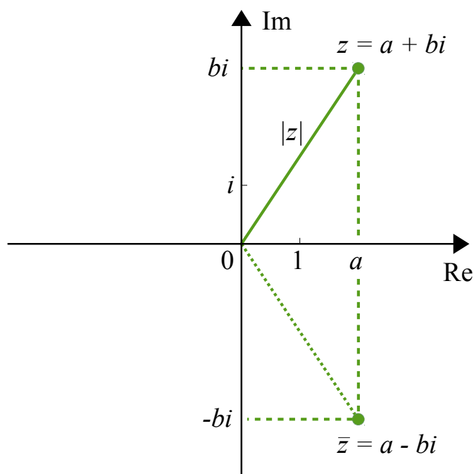
Rysunek 2.1: Interpretacja geometryczna liczby zespolonej.
