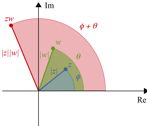
Rysunek 2.4: Iloczyn liczb zespolonych
