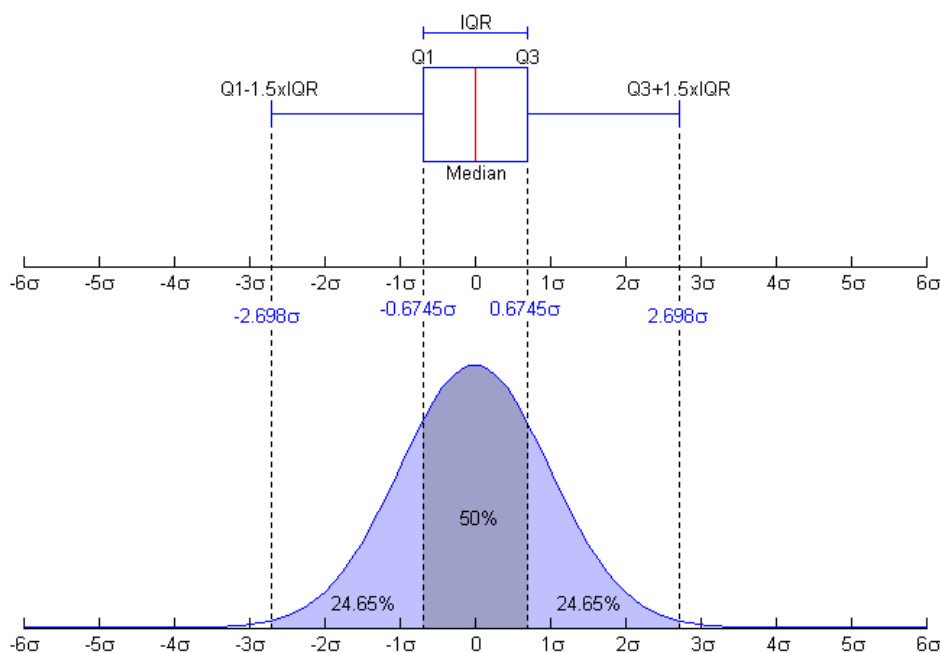
Rysunek 2.1: Elementy wykresu pudełkowego na przykładzie rozkładu normalnego: mediana, pierwszy i trzeci kwartył ( Q1 , Q3 ), zakres międzykwartyłowy ( IQR ). Wartości poza tzw. wąsami (przedziałem [Q1 - 1.5 \cdot IQR, Q3 + 1.5 \cdot IQR] ) są nazywane obserwacjami odstającymi (ang. outliers) i w środowisku R są rysowane jako pojedyncze punkty. Źródło rysunku: http://en.wikipedia.org .
